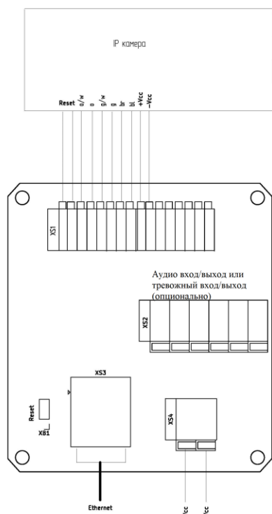
Рисунок Б1 – Подключение IP видеокмеры с питанием 12 VDC
