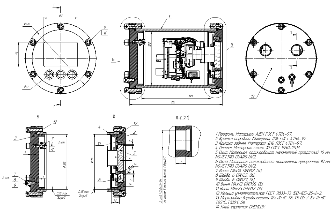
Рисунок А3 – Чертеж безопасности
