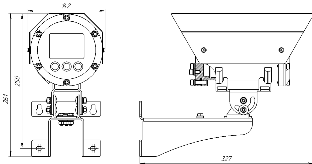
Рисунок А1 – Габаритные размеры видеокамеры АйТек ПРО H10-Exd
