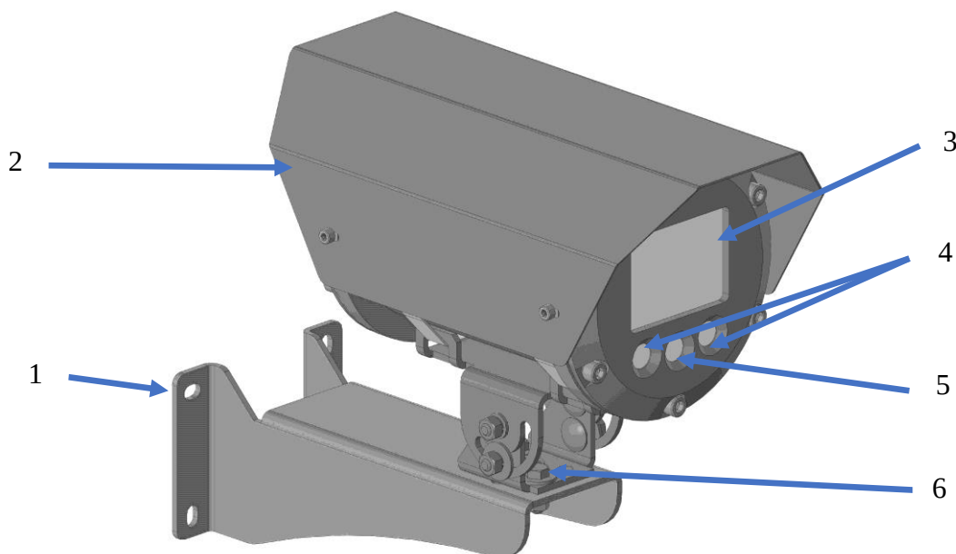
Рисунок 1 – Внешний вид видеокамеры АйТек ПРО Н10-Exd
