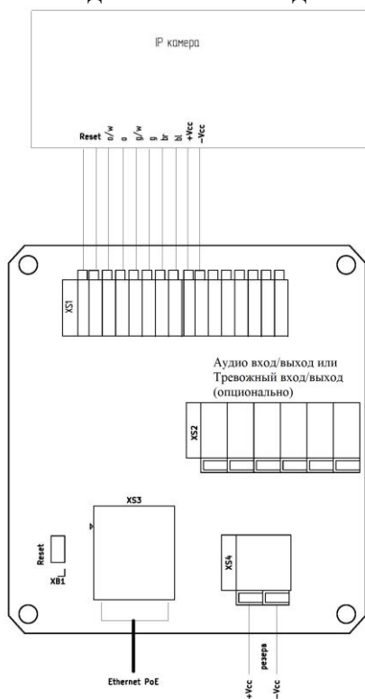
Рисунок Б2 – Подключение IP видеокмеры с питанием PoE
