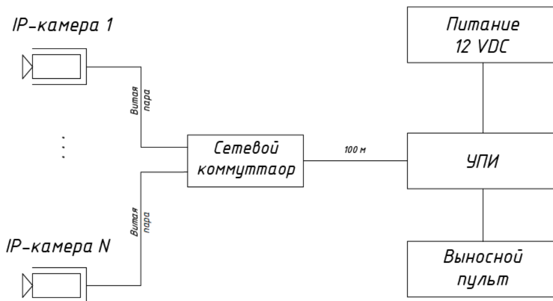
Рисунок Б1 – Схема подключения УПИ с встроенным регистратором
